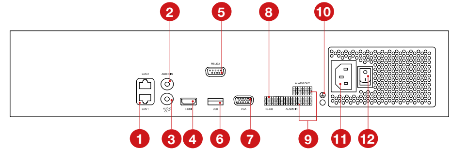
Рисунок 3.16 Задняя панель IP регистраторов (корпус под 4 HDD).
